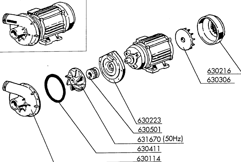
100361 (1.5kW 400V 50Hz)
