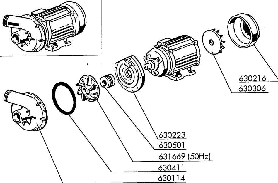
100703 (1.1kW 400V 50Hz)
